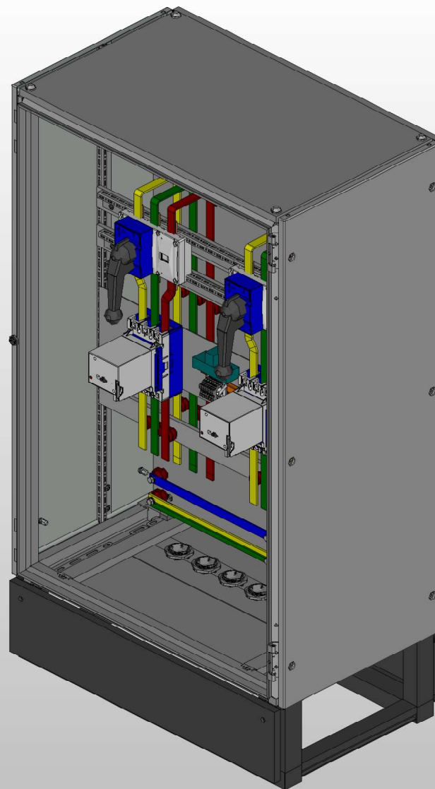
Вид без двери
