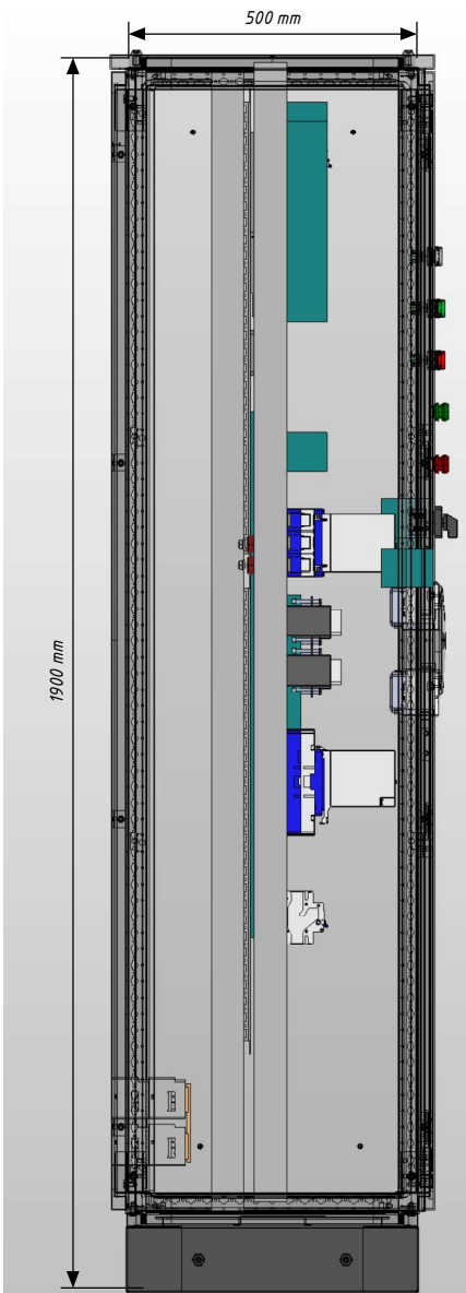
Вид слева
