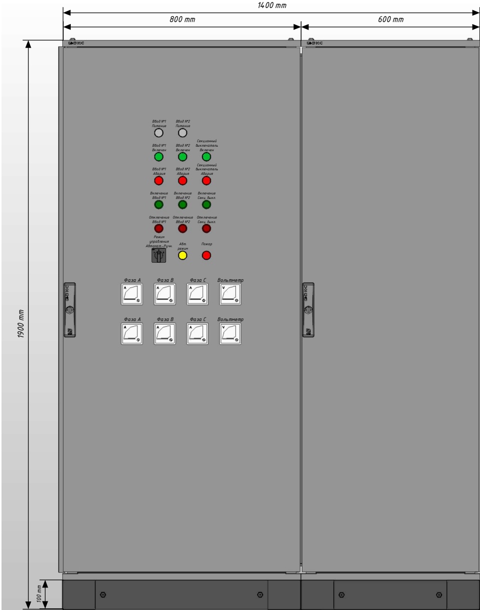
Вид спереди с дверями
