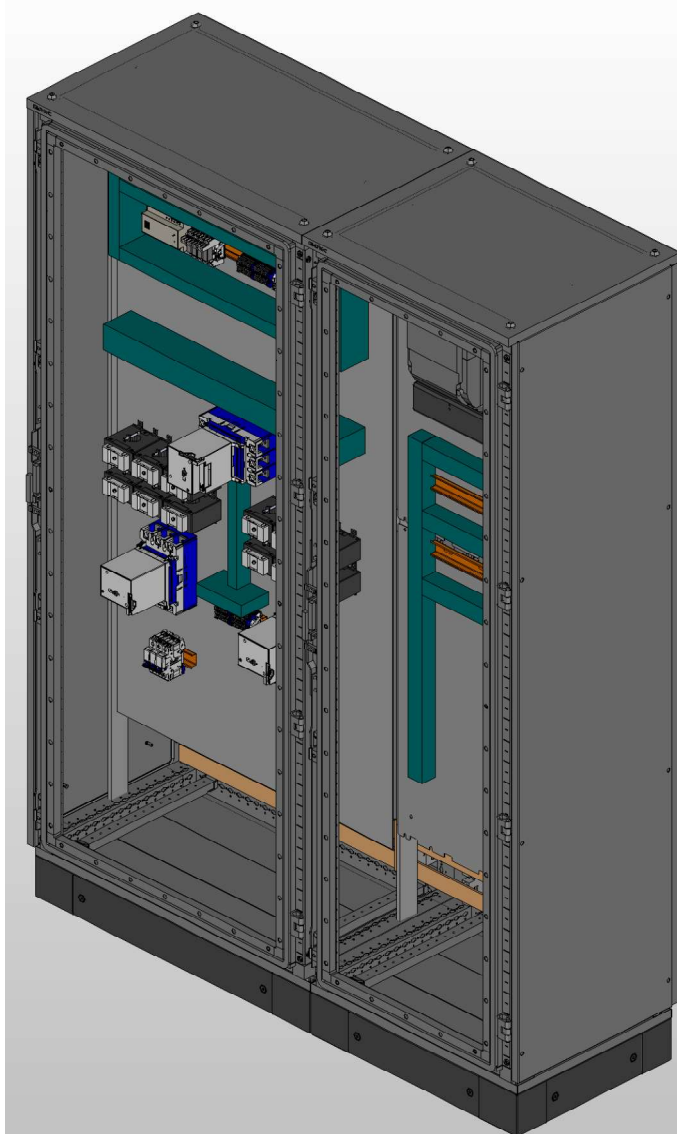
Вид спереди без дверей и с дверями (изометрия)
