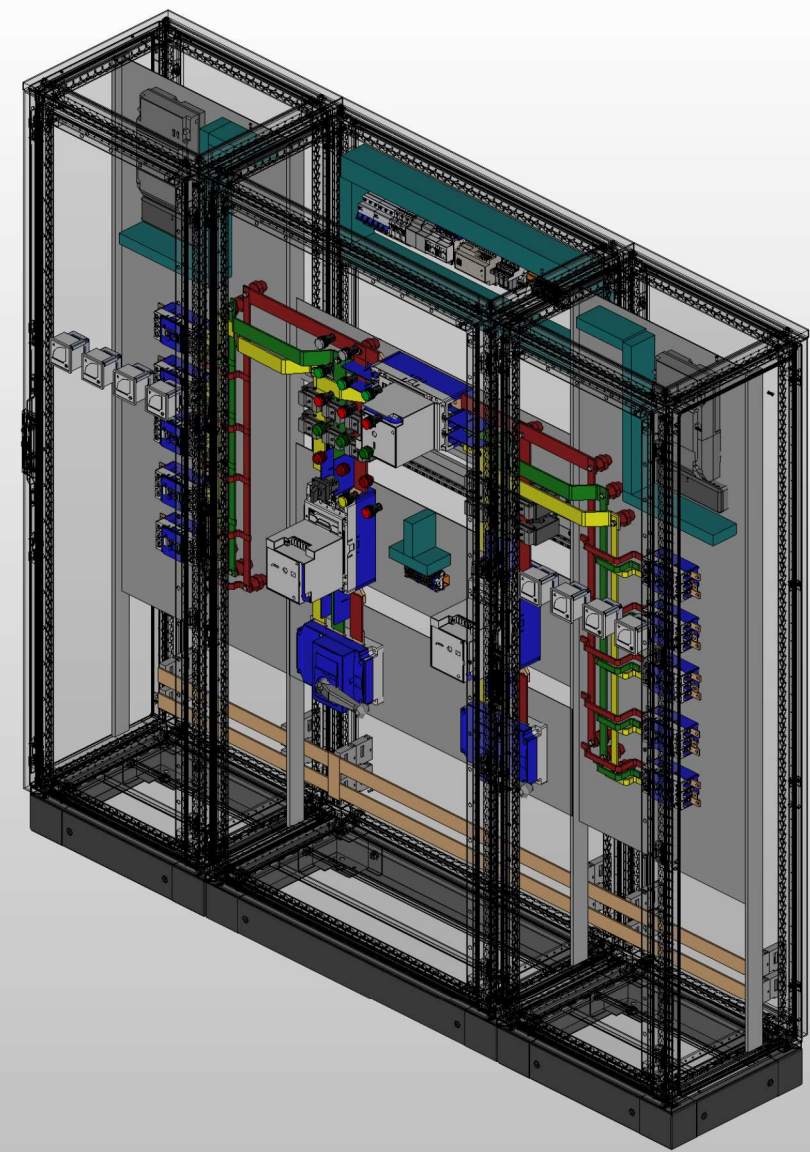
Вид спереди с дверями (изометрия)
